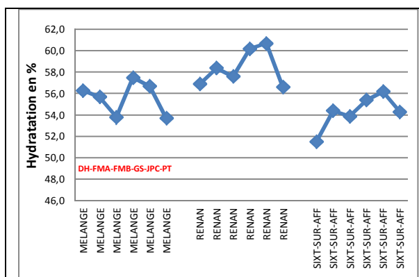
Figure 7 : Hydratation de la pâte au Farinographe
